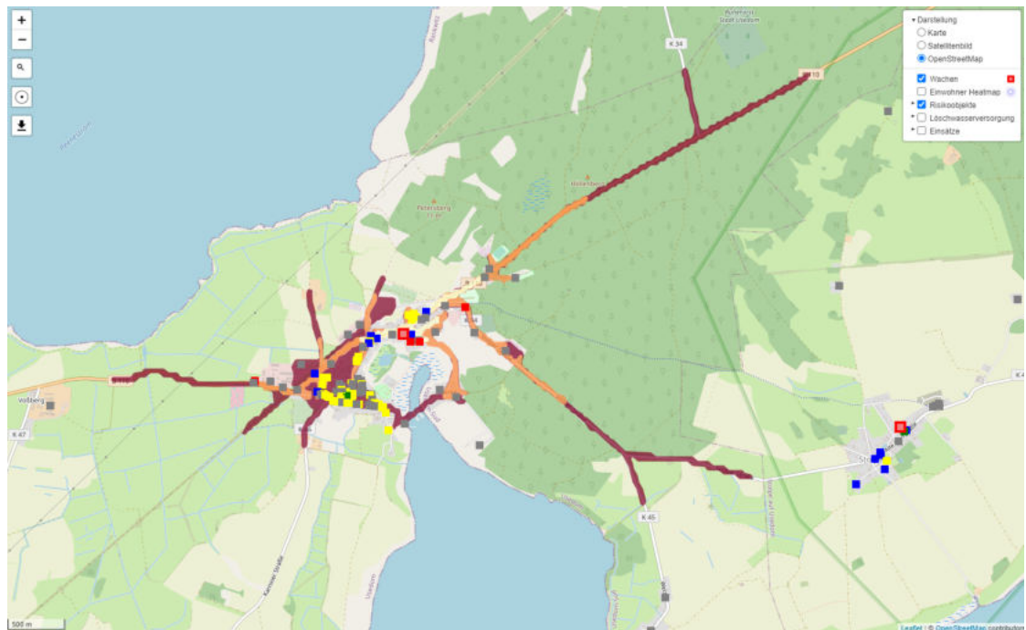
Abbildung G.5 – Modellierter Abdeckungsgrad der Primäreinheit der Gemeindefeuerwehr Usedom für 3 min Fahrzeit (Isochrone mit 3 min-Raster); Abdeckungsgrad in Bezug auf das Gemeindegebiet = 66 %
