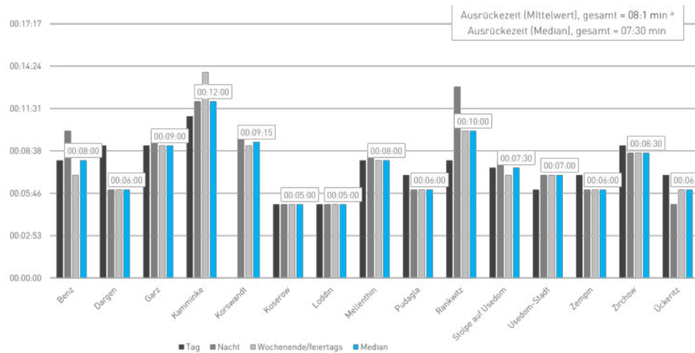
Abbildung G.4 – Statistische Ausrückezeit der Primäreinheit der Gemeindefeuerwehr Usedom im Amtsvergleich (Betrachtungszeitraum 01/2018 – 09/2021)
