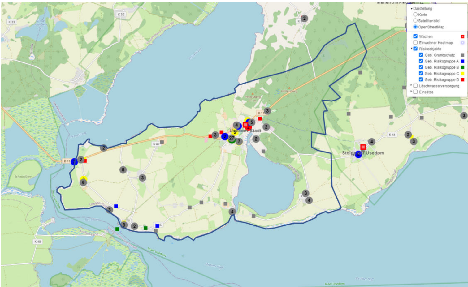
Abbildung G.1 – Gesamtübersicht der Verkehrsinfrastruktur der Stadt Usedom einschließlich Kartierung der Risikooobjekte (Kategorien Grundschatz, A - D )
