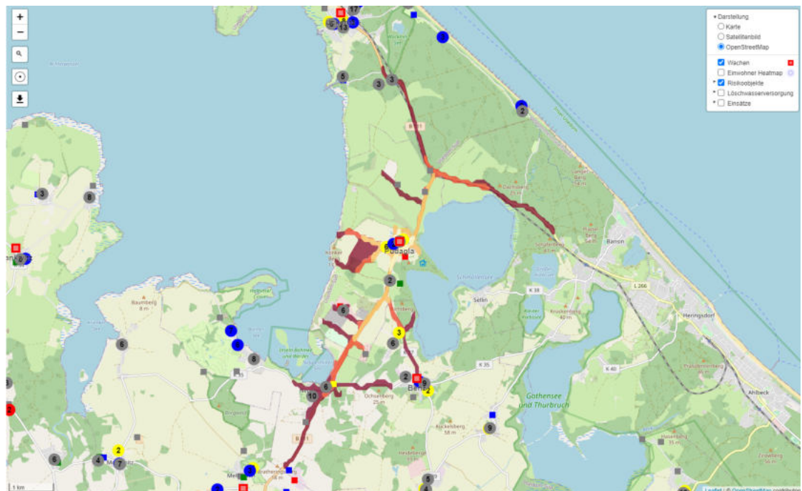
Abbildung G.5 – Modellierter Abdeckungsgrad der Primäreinheit der Gemeindefeuerwehr Pudagla für 4 min Fahrzeit (Isochrone mit 4 min-Raster); Abdeckungsgrad in Bezug auf das Gemeindegebiet = 97 %
