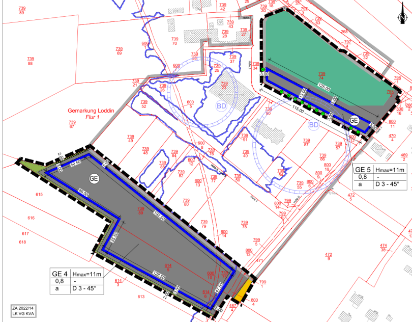
Planzeichnung (Teil A)
