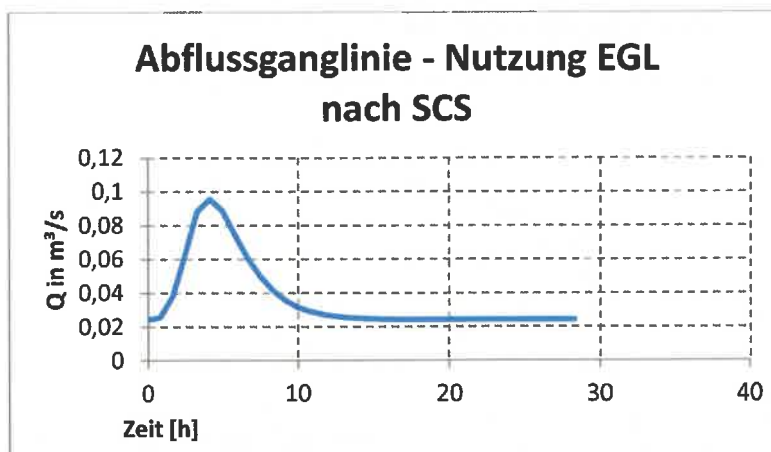
Abbildung 13: Abflussganglinie für Modellregen mit 2-jährigem Wiederkehrintervall
