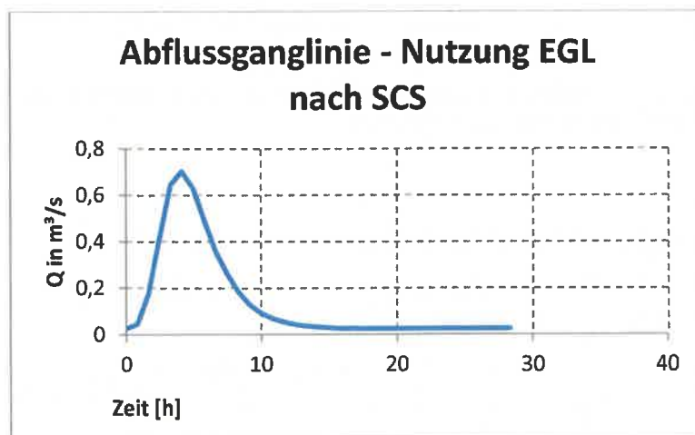
Abbildung 14: Abflussganglinie für Modellregen mit 50-jährigem Wiederkehrintervall
