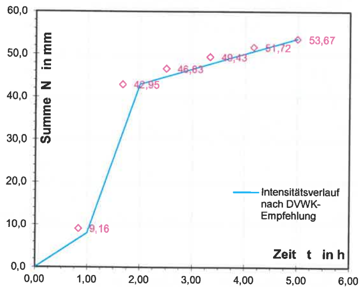
Abbildung 12: Intensitätsverlauf Niederschlag nach Kostra DWD 2000 für Modellregen mit 50-jährigem Wiederkehrintervall
