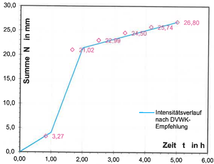
Abbildung 11: Intensitätsverlauf Niederschlag nach Kostra DWD 2000 für Modellregen mit 2-jährigem Wiederkehrintervall
