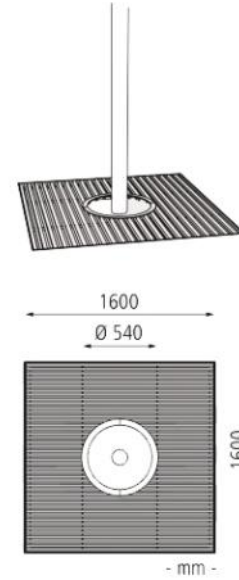
Technische Zeichnung
