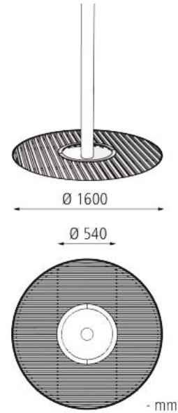
Technische Zeichnung
