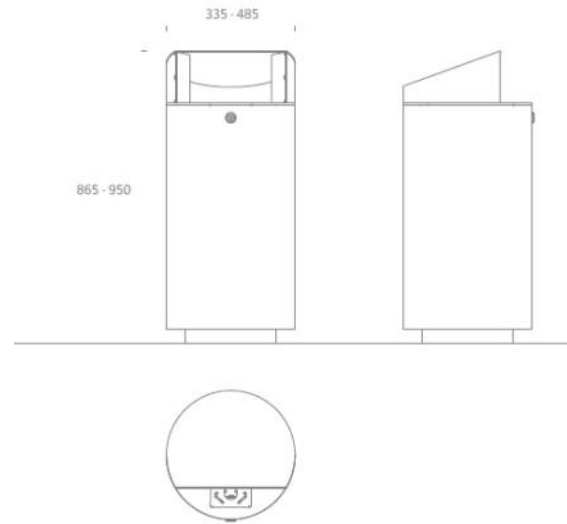
Technische Zeichnung
