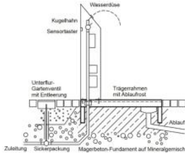
Technische Zeichnung
