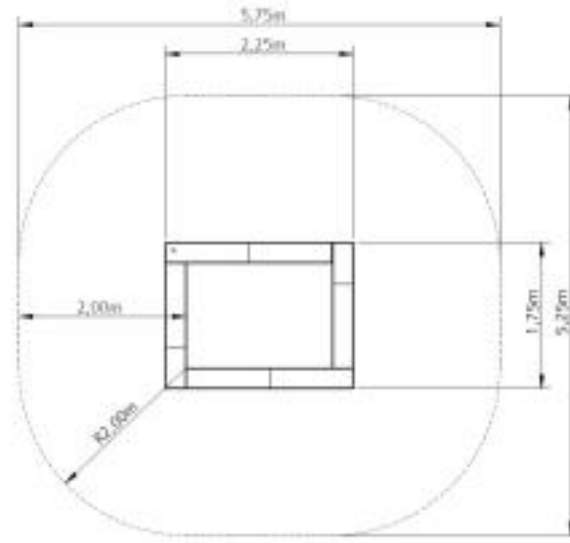
Technische Zeichnung
