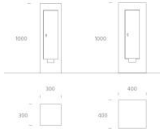
Technische Zeichnung
