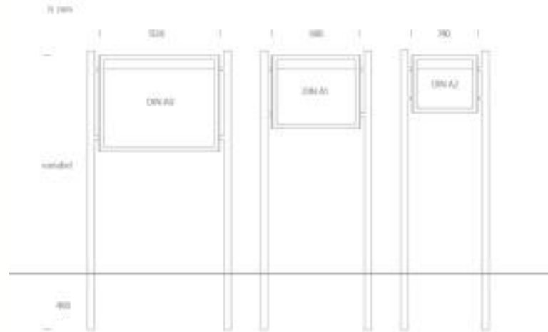
Technische Zeichnung
