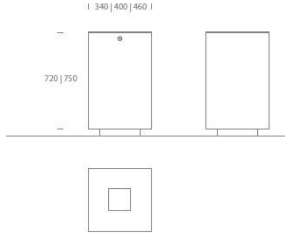
Technische Zeichnung
