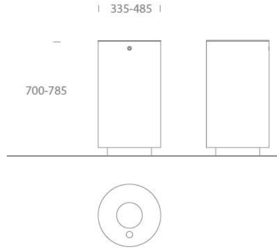
Technische Zeichnung
