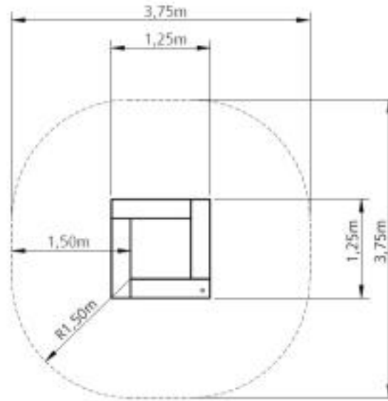
Technische Zeichnung
