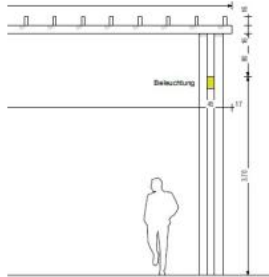
Technische Zeichnung
