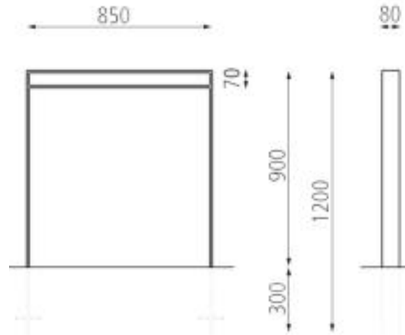
Technische Zeichnung
