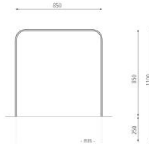
Technische Zeichnung
